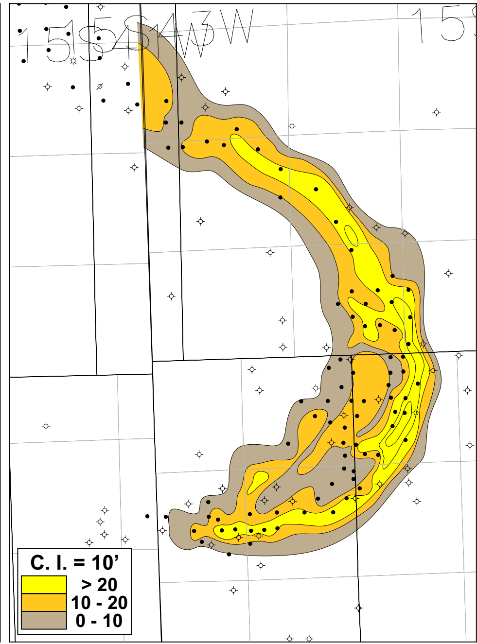
Stockholm Net Sand Isopach Map
